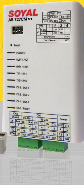
串列設備連網伺服器 AR-727CM
